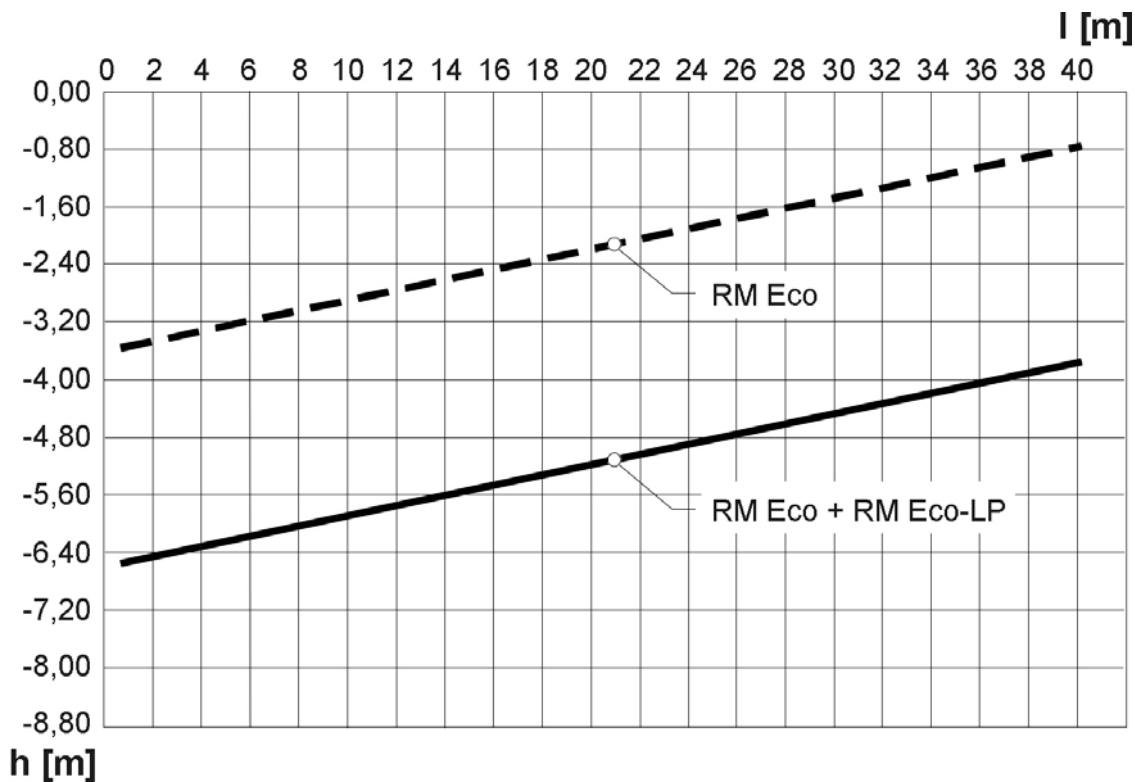
Ansaugkennlinie mit und ohne Ladepumpe RM Eco-LP
