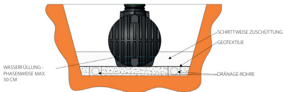
Abbildung 7: Behältereinbau in schlecht durchlässige Bodenflächen
