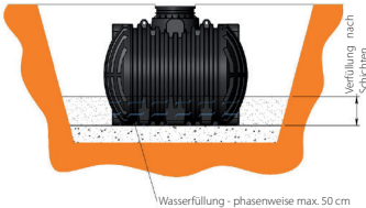
Abbildung 2: Aufstellung und Zuschüttung des Behälters
