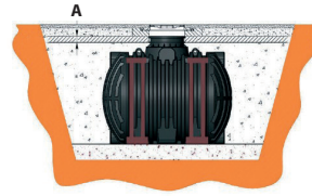
Abbildung 10: Behältereinbau mit Verschalungs- und Stützsäulentragwerk
