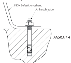
Abbildung 5: Detaillierte grafische Darstellung der Befestigung mit Inoxband
