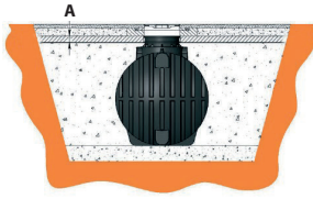
Abbildung 9: Behältereinbau unterhalb befahrbarer Flächen
