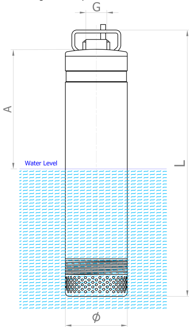
Abbildung 4: Minimale Eintauchtiefe iDiver Inox
