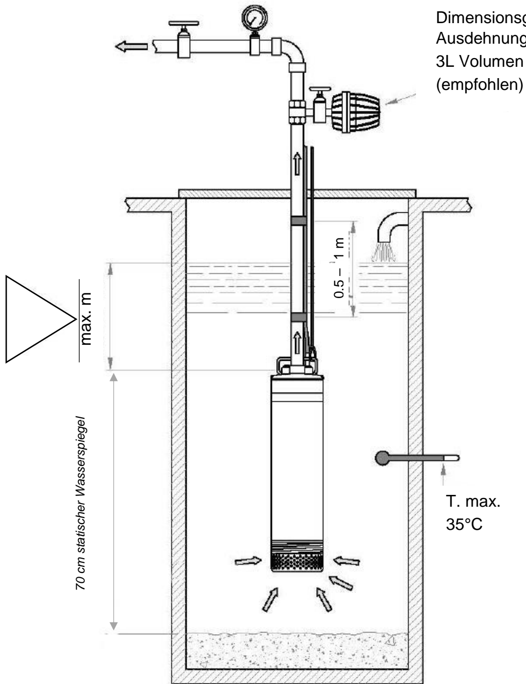
Abbildung 1: Einbauvorschriften iDiver Inox
