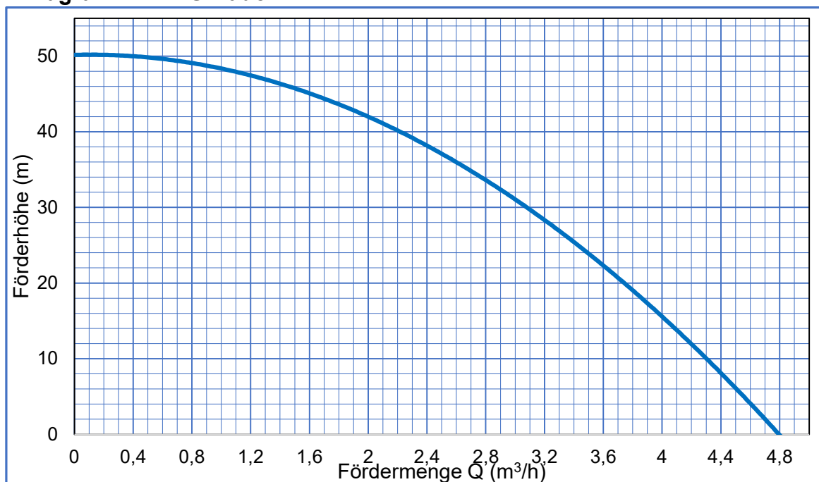
Diagramm 3.4.1.1 Q / H Diagramm TWTS-Hader
